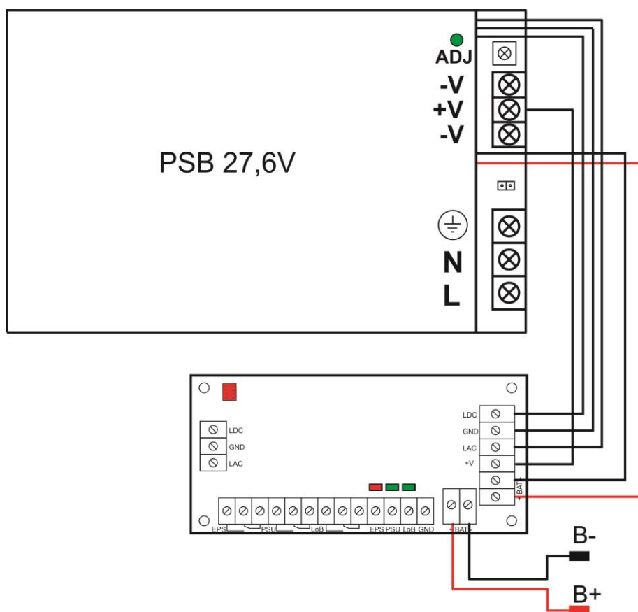
Rys.2 Schemat podłączenia modułu do zasilacza PSB.
